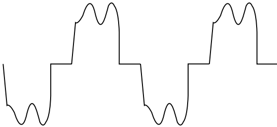
Iligne réseau consommé par un redresseur triphasé.
