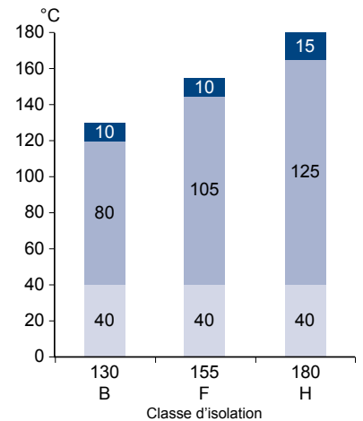
Échauffement ( \Delta T^* ) et températures maximales des points chauds ( T_{max} ) selon les classes d'isolation (norme CEI 60034 - 1).
