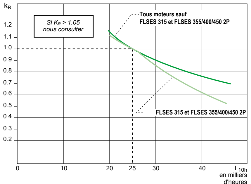
Évolution de la durée de vie L_{10h} des roulements en fonction du coefficient de charge radiale k_R pour les montages standard.
