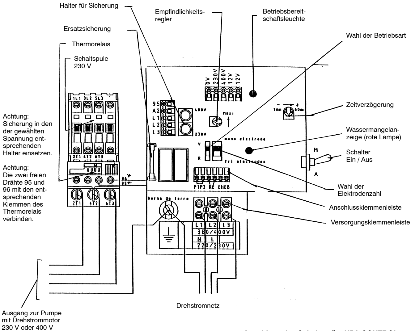
Anschluss des Schaltgeräts UPA CONTROL an ein Drehstromnetz 230 V oder 400 V
