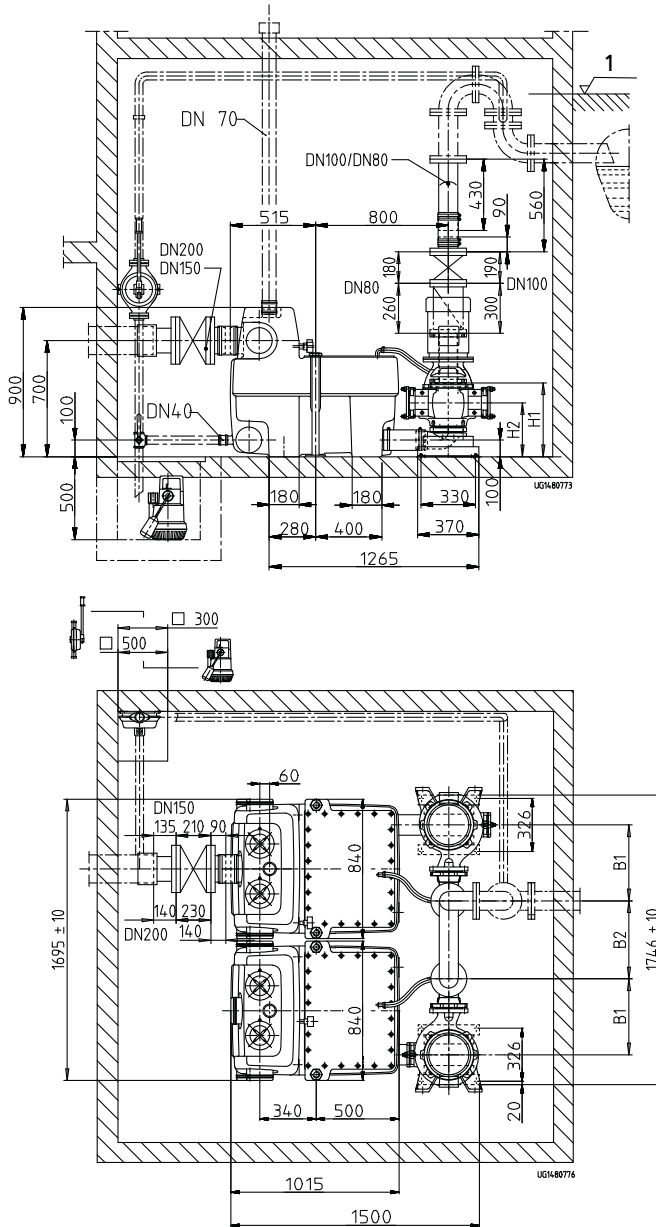
III. 5: Cotes d'installation Compacta UZ, ZF, ZK 20.900 D à 67.900 D [mm]
