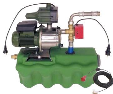
CENTRALE DE PILOTAGE avec flotteur - Code 355002
