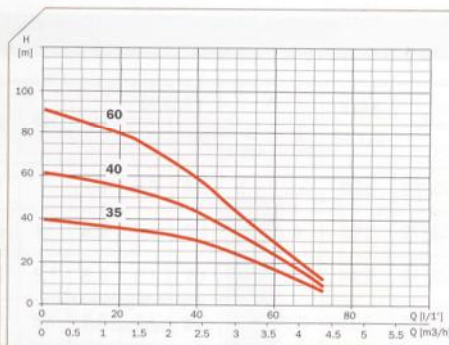
Courbes hydrauliques
