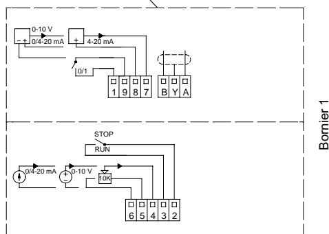
Fig. 27 Schéma de câblage en monophasé des TPE
