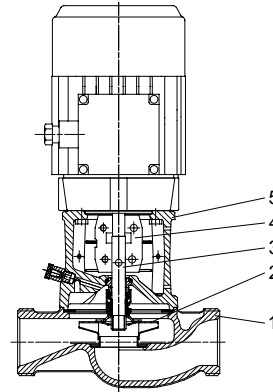
Fig. 3 Dessin en coupe des TP série 100 (avec raccord-union)
