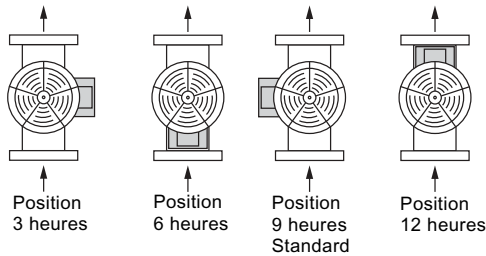
Fig. 23 Positions possibles de la boîte à bornes
