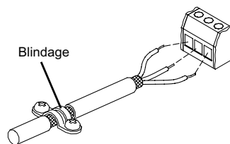
Fig. 25 Connexion du câble de Marche/arrêt externe des TPE, TPED
