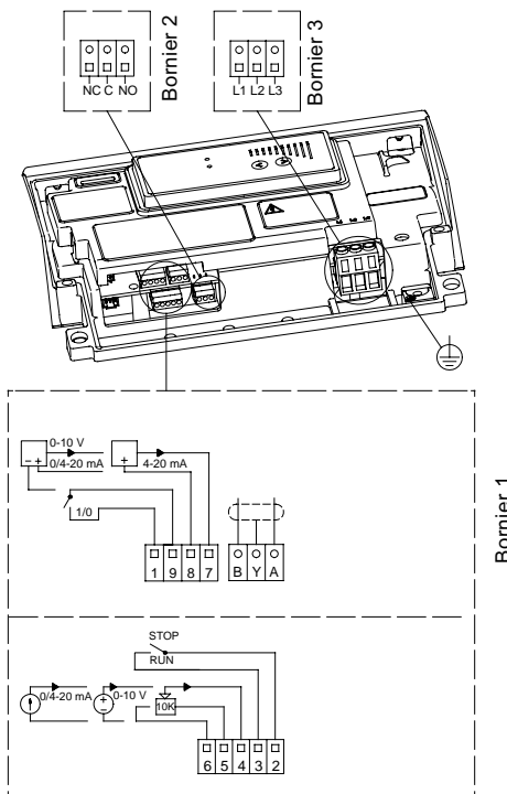
Fig. 28 Schéma de câblage en triphasé des TPE
