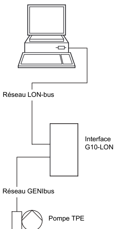
Fig. 11 Structure d'un poste central de télégestion
