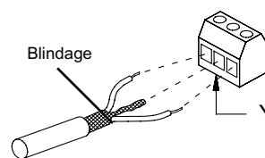
Fig. 26 Connexion bus des TPE, TPED
