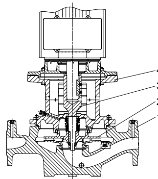
Fig. 6 Dessin en coupe des pompes TP série 300
