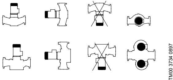
Fig. 16 Installation des pompes équipées de moteurs jusqu'à 7,5 kW inclus
