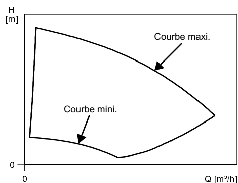
Fig. 14 Courbes de performances mini et maxi
