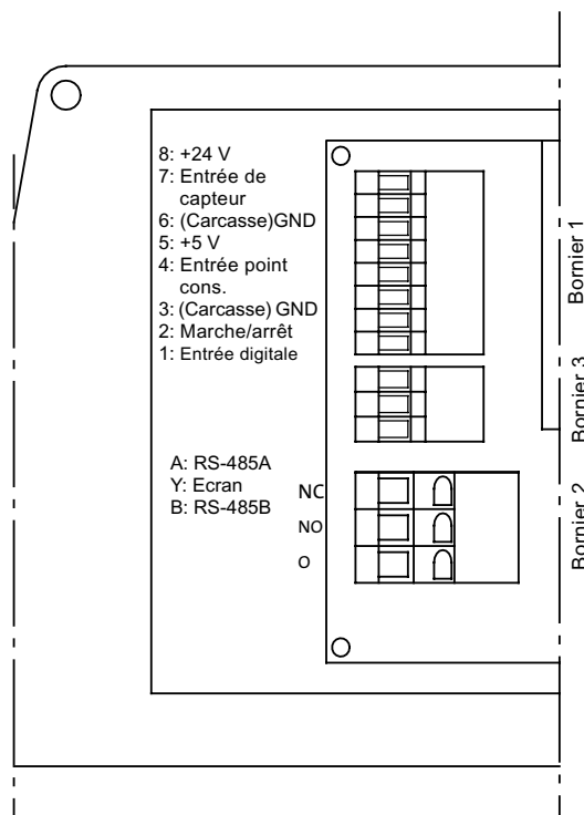
Fig. 29 Schéma de câblage en triphasé des TPE, TPED
