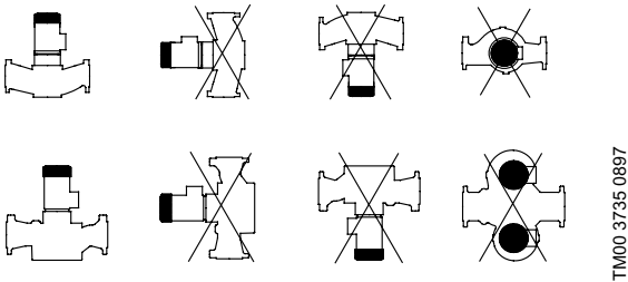
Fig. 17 Installation des pompes équipées de moteurs supérieurs à 7,5 kW
