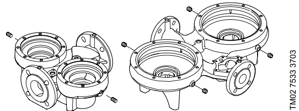
Fig. 18 Prises pour montage des purgeurs d'air automatiques TP série 200 et TP série 300
