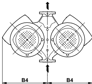
Fig. 24 Positions de la boîte des pompes TPED
