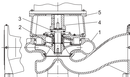
Fig. 8 Dessin en coupe des pompes TP série 400
