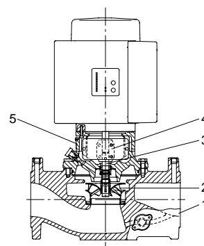
Fig. 4 Dessin en coupe des pompes monophasées TPE série 200 (modèle avec bride)
