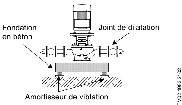
Fig. 20 Fondation de la pompe TP
