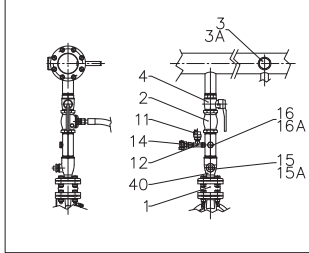
VERSION AVEC VANNE FILETÉE
