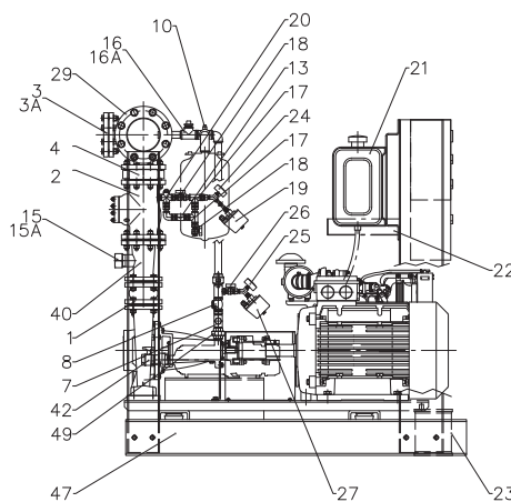
VERSION AVEC VANNE BRIDÉE
